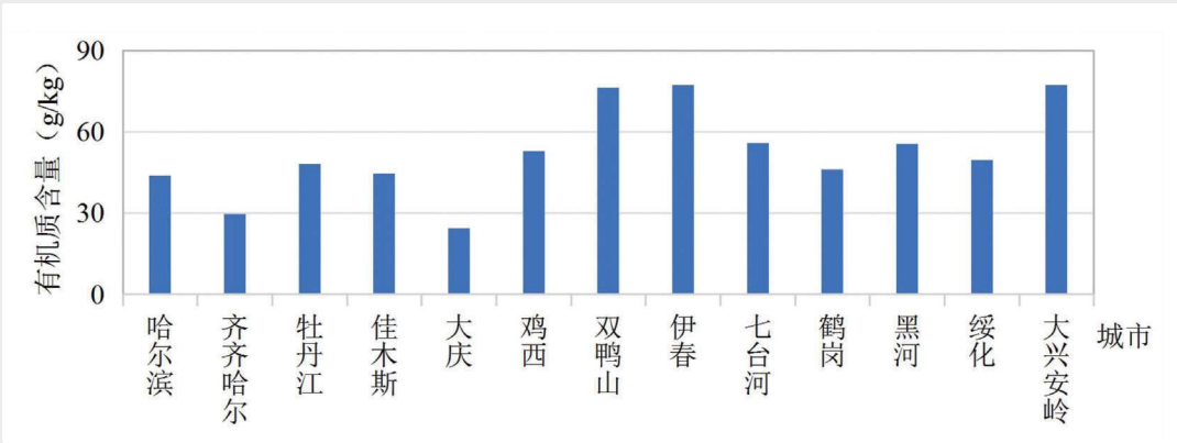
全省土壤有机质示意图
